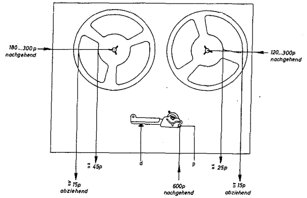
Abb. 12 Mechanische Meßpunkte
