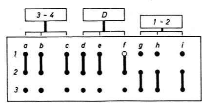
Spurumschalter (Spur, 1-2 "gedrückt") TRACK SWITCH CONNECTEUR DE PISTES
